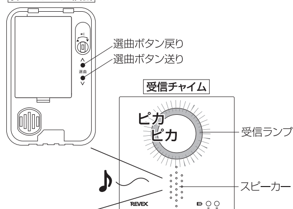
押しボタン送信機
